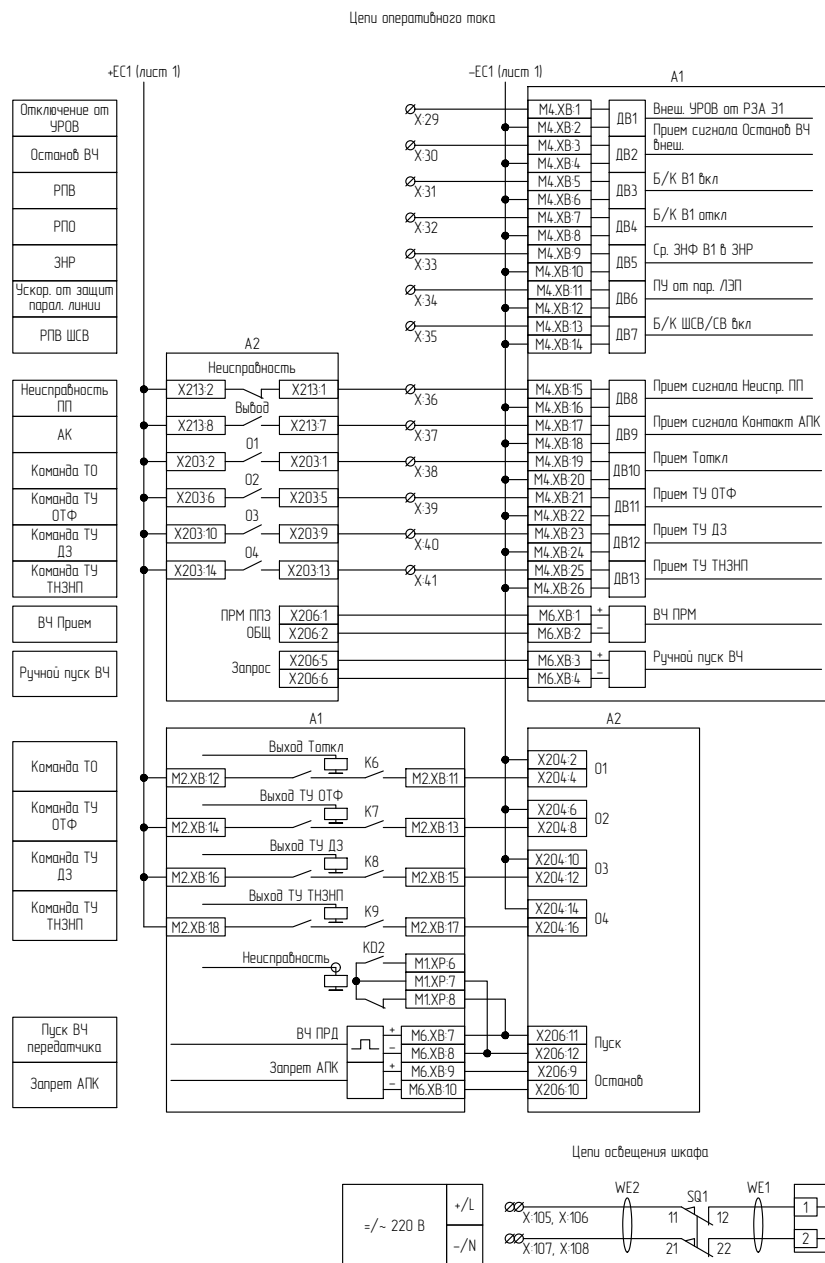
Рисунок В.2 – Схема электрическая принципиальная (часть 2)
